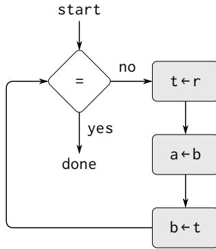
Figure 5.2: GCD マシンのコントローラ
