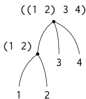
Figure 2.6: 木として見た Figure 2.5 のリスト構造
